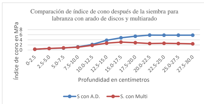
Figura 2. Comportamiento del índice de cono en las diferentes labranzas. a) Ic después de la siembra y cosecha con preparación de suelo con arado de discos, b) comparación del Ic después de la siembra para ambas preparaciones del suelo. S-siembra y C-cosecha. Toluca, México, 2018-2019.
