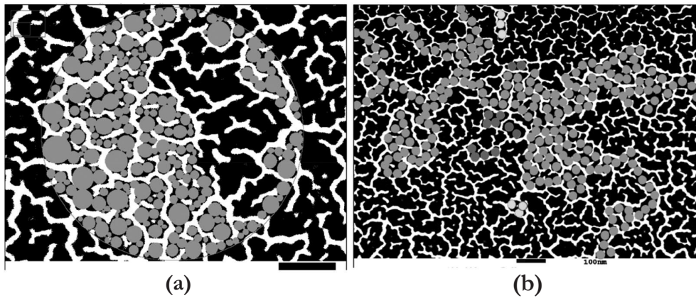
Figura 6. Oro depositado en silicio por un tiempo de 11 minutos. En ambas figuras, la barra densa color negro define la escala a 100 nm. (a) Esquematación del procedimiento usado para determinar la fracción de llenado superficial metálica, se muestra un llenado parcial del área seleccionada. (b) Esquematación de caminos de conducción eléctrica. La trayectoria trazada en color gris es no cerrada, con poco más de 200 círculos contiguos y de diámetro igual a 30 nm: la extensión total de la trayectoria bien podría ser cercana a los diez micrómetros. Con distintos colores se muestran los pocos casos presentes de trayectorias cerradas, y con extensiones aproximadas de 60 y 100 nm
