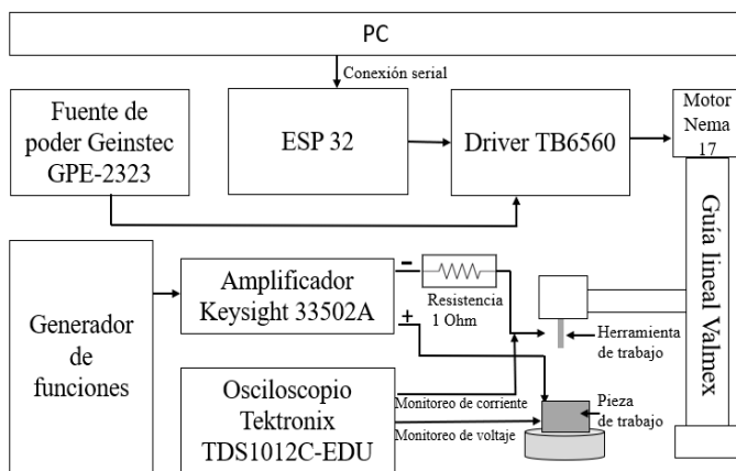
Fig. 1. Diagrama a bloques del prototipo ECM
