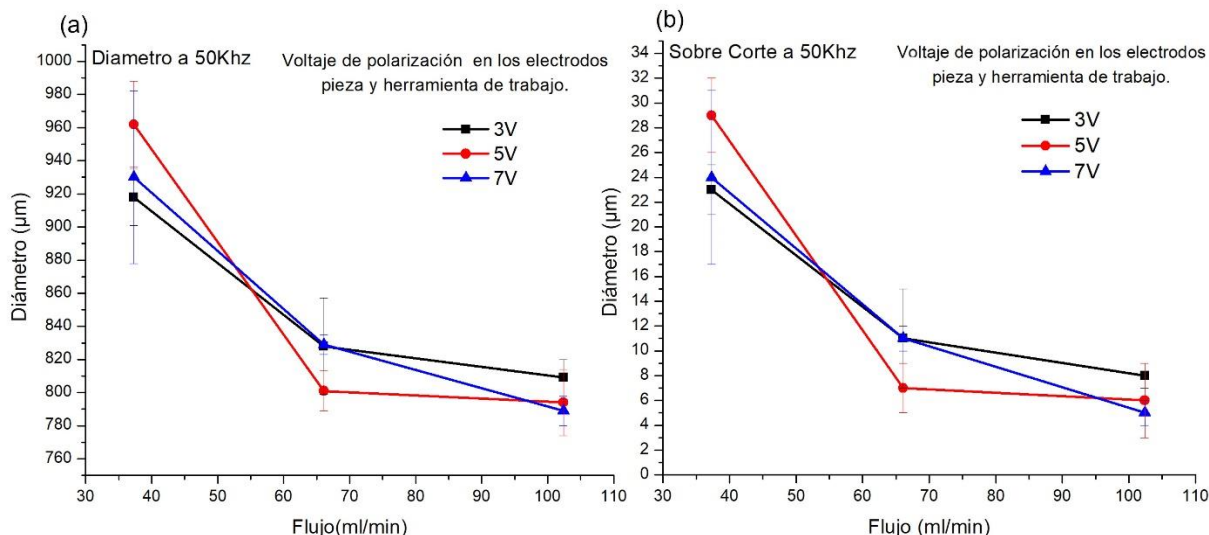
Fig.7. Graficas de comparación del diámetro (a) y sobre corte (b) a 50 kHz.
