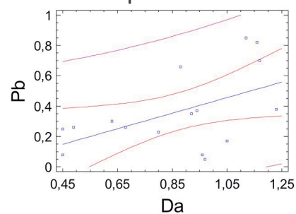
Figura 3. Correlación Pb-Densidad Aparente
