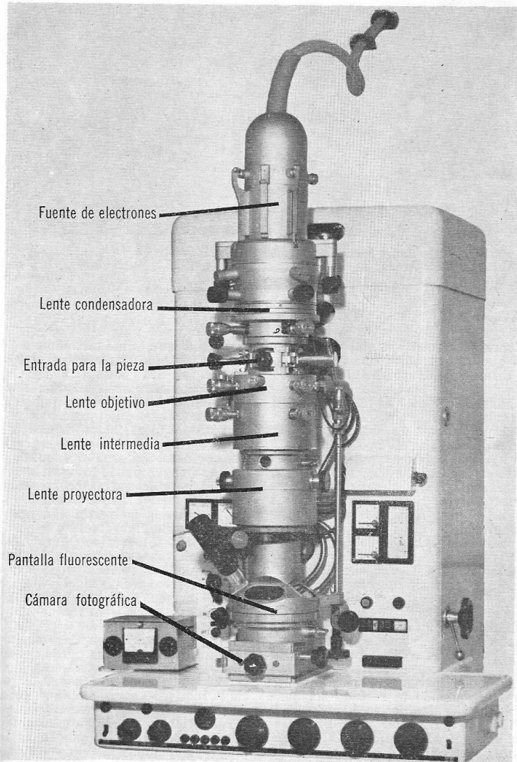
FIG. 4-9. Microscopio electrónico Siemens.
