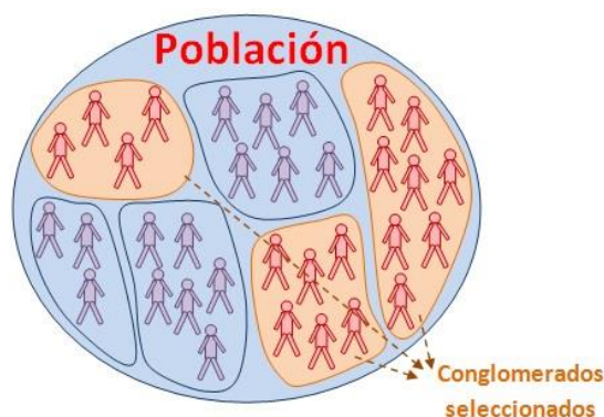
Figura 24. Muestra por conglomerados
