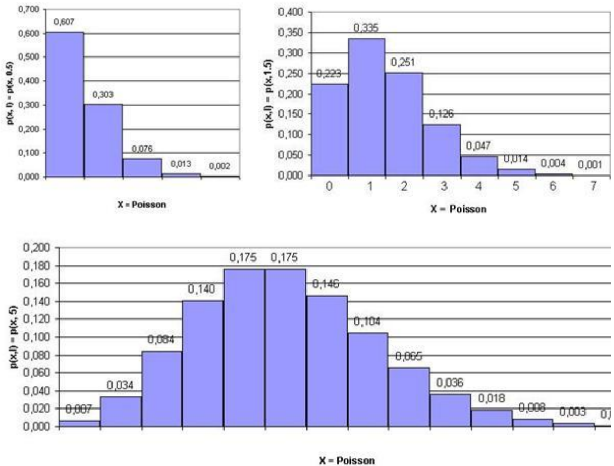
Figura 16. Gráfico de distribución de Poisson
