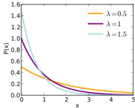
Figura 18. Gráfico distribución Exponencial
