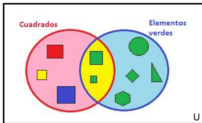
Figura 7. Diagrama de Venn
