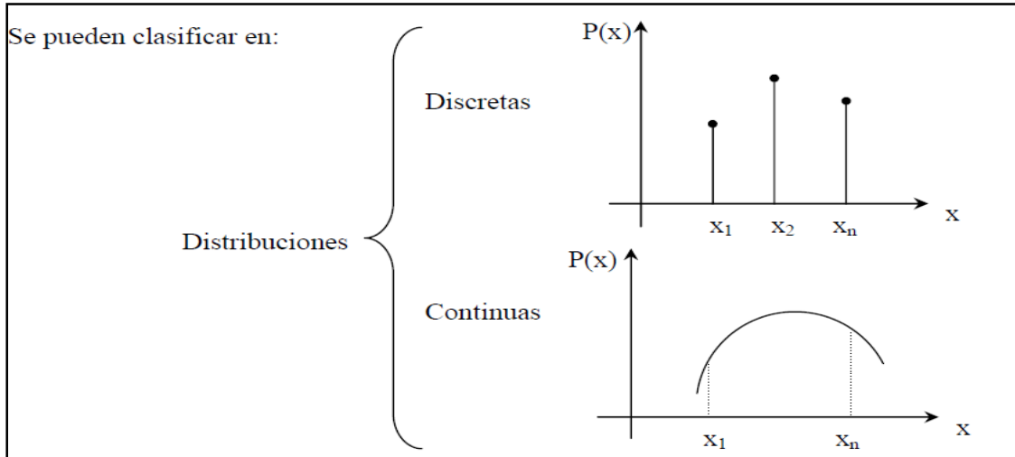
FIGURA 10. Clasificación de distribuciones de probabilidad
