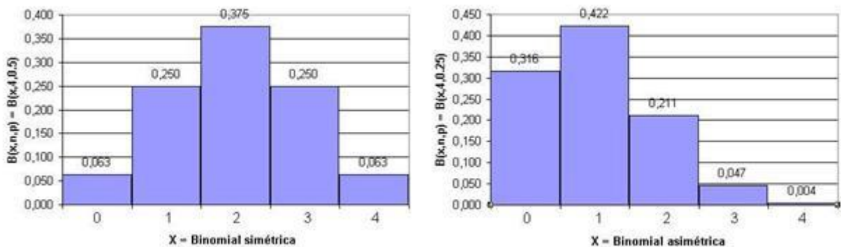
Figura 14. Gráfica distribución de binomial
