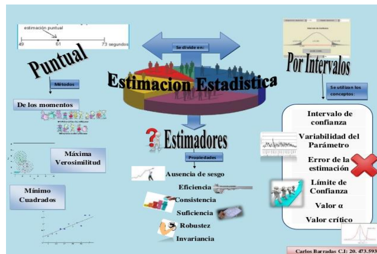
Figura 36. Estimación puntual y por intervalo
