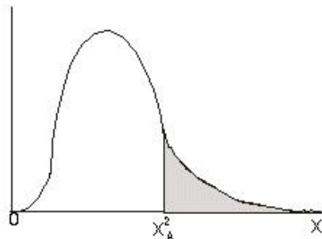
Figura 30. Distribución muestral de varianza Fuente: imagen recuperada de www.google.com.mx
