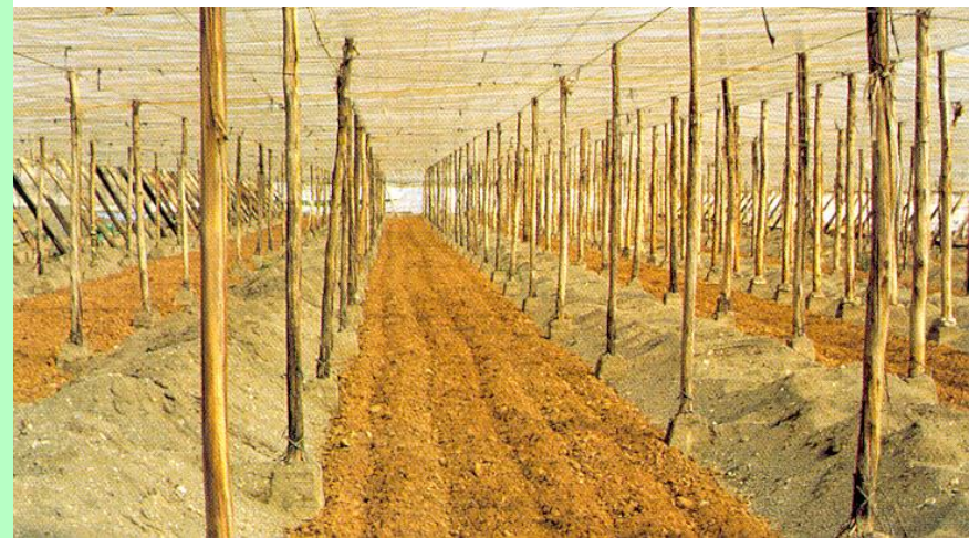
Esquema de un enarenado
