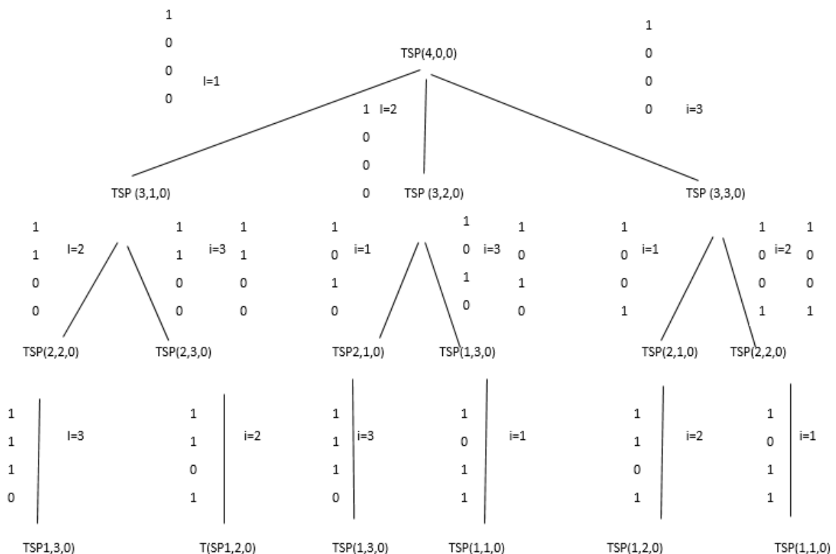
Figura 8.5 Uso del vector m .
