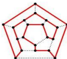
Fig. 9.7 Ejemplo de un ciclo Hamiltoniano.
