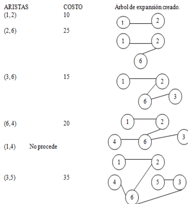
Fig. 7.5 Solución paso a paso del árbol de expansión mínima.
