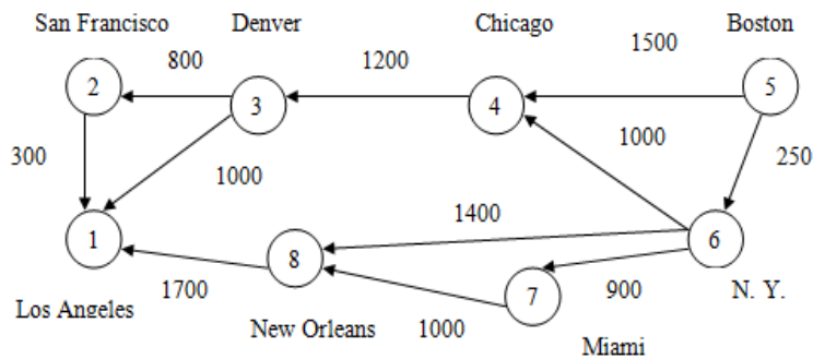
Fig. 7.7 Un ejemplo para el trayecto más corto.
