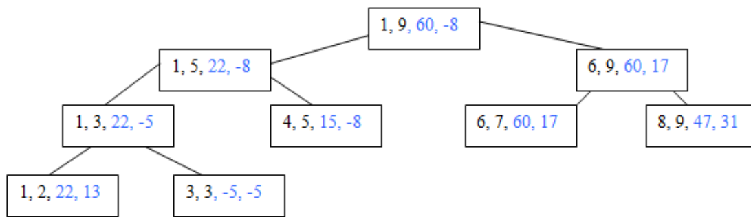
Fig. 6.1 Árbol recursivo con el algoritmo MaxMin.
