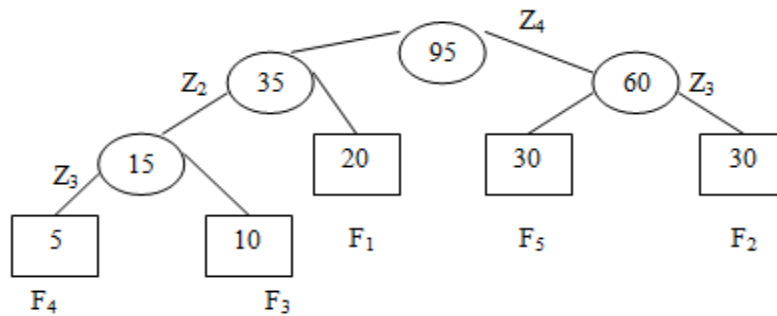
Fig. 7.1 Patrón óptimo de concatenación.
