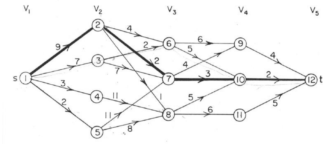
Fig. 8.1 Gráfica de 5 etapas.
