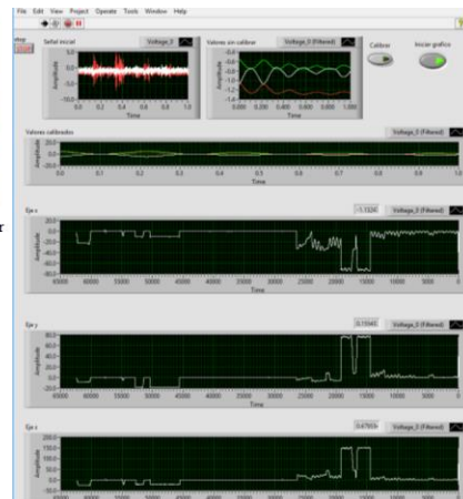
Figura 7 Interfaz de LabView para monitoreo del dinamómetro KISTLER 5010B.
