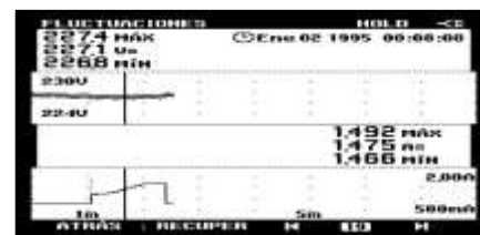
Figura 5. Ejemplo de fluctuaciones de voltaje y corriente registradas en el arranque y apagado de una lámpara.
