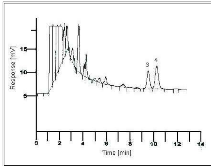
Figura 3. Inyección de una mezcla de cloro de 1 mg/L disuelto en un buffer de fosfatos (pH 7), 50 µg/L de m-clorofenol. Tiempo de contacto 30 minutos.
