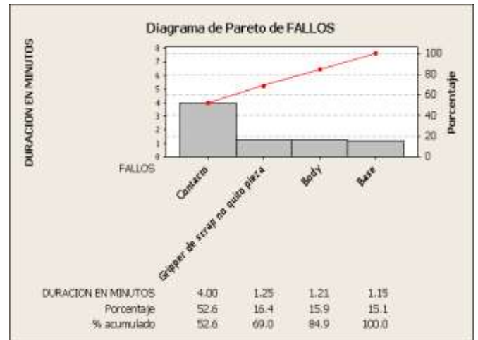
figura. 3. Duración de fallos (en minutos)
