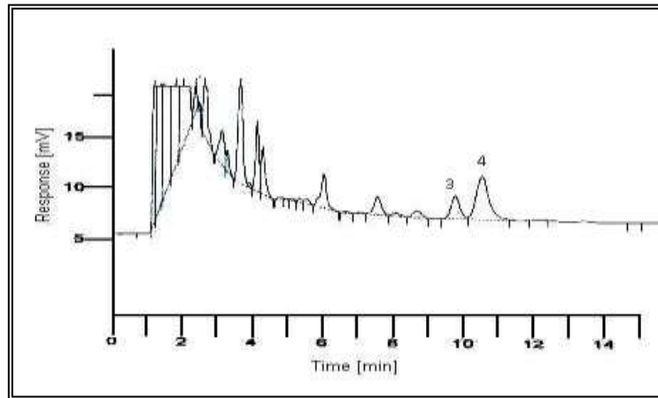
Figura 2. Inyección de una mezcla de cloro de 1 mg/L disuelto en un buffer de fosfatos (pH 7), 50 µg/L de m-clorofenol. Tiempo de contacto 10 minutos.
