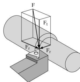
Figura 2 Componentes de la fuerza de corte F ; F_t fuerza tangencial, F_a fuerza de avance y F_r fuerza radial.
